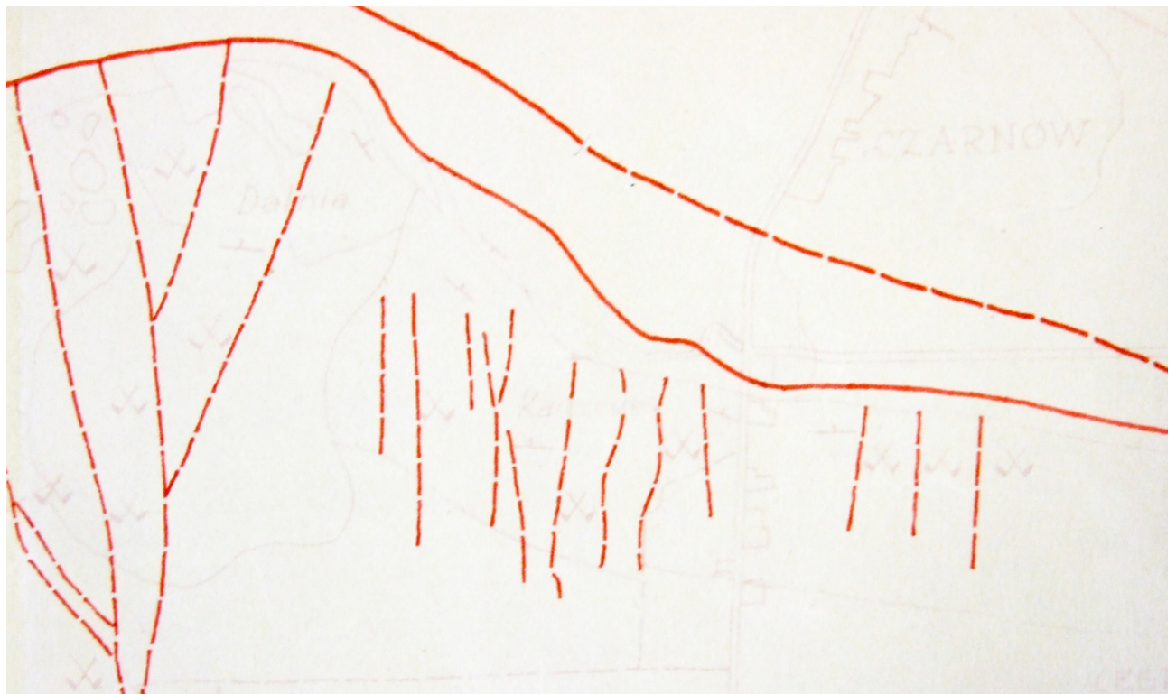
Ryc. 3. Szkic geologiczny rejonu południowego skrzydła synkliny kieleckiej, rys. J. Czarnocki (fragment), WAP - ukazujący linie tektoniczne związane ze starymi robotami górnymi rejonu Karczówki i Dalni
